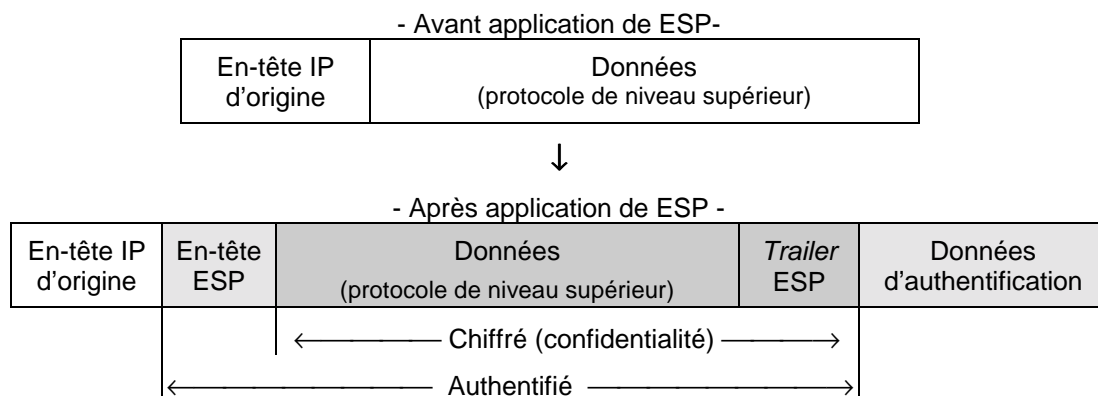
- Figure 8. Position de ESP en mode transport (IPv4) -
